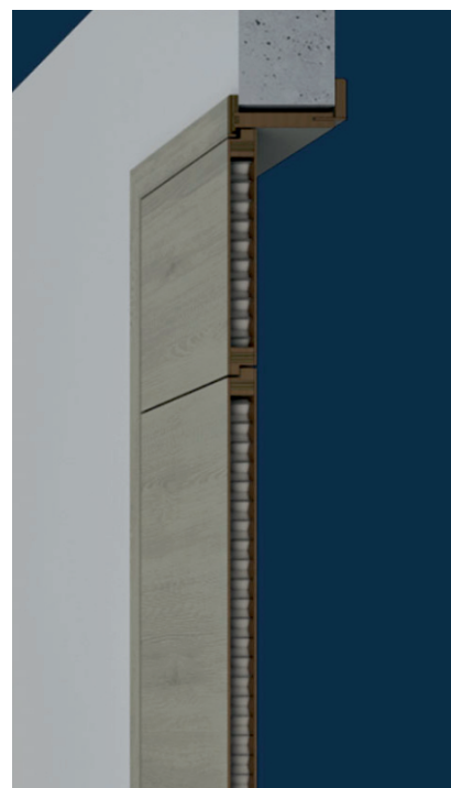
Tokbanyíló fix blendével
