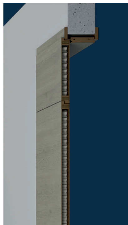
Falcnélküli osztott blendével
