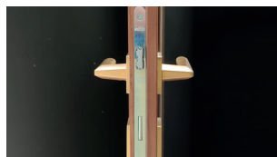
Az ajtólap 40 mm vasatagságú, PZ vagy WC zár kialakítással
