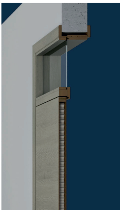
Falc nélküli tokosztós felülvilágítóval
