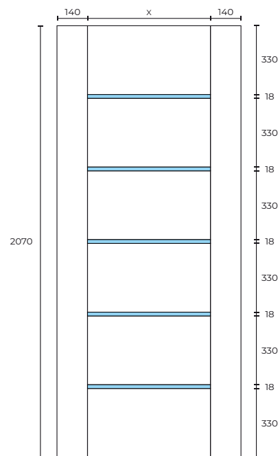
Atlanta ajtómodell méretei
