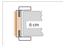
Mozgó borítás fedérének vágásával 6 cm-es falavas- tagságra igazítható a tok
