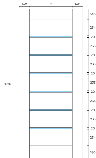
Sonata ajtómodell méretei
