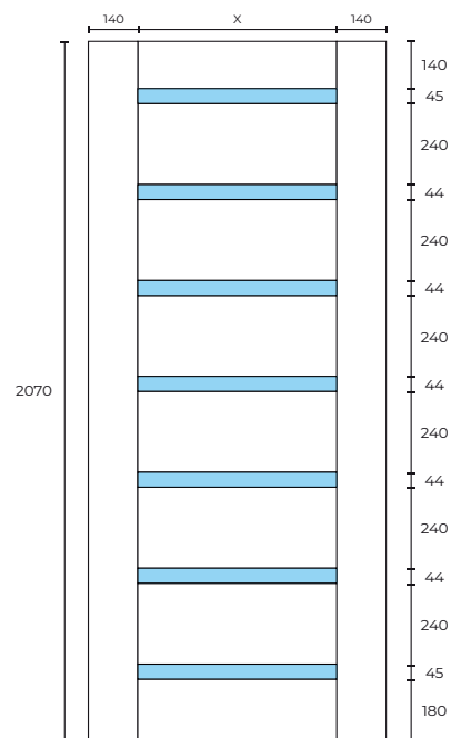
Torino ajtómodell méretei
