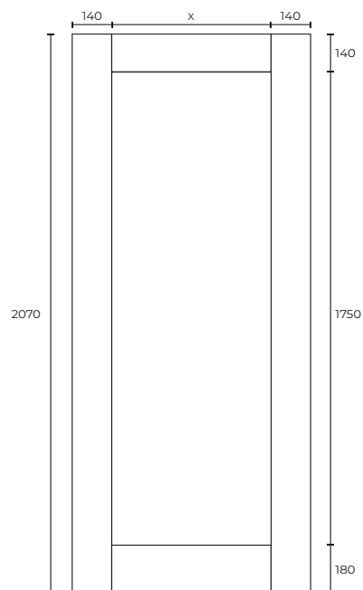
Lizbona ajtómodell méretei
