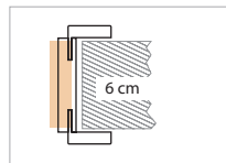
Mozgó borítás vágásával 6 cm-es falvastagságra igazítható a tok/panel tok
