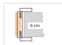
Mozgó borítás vágásával 6 cm-es falvastagságra igazítható a tok/panel tok
