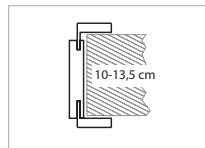
Széles állíthatóságú átfogó tok
