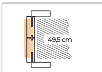
Toktoldással akár 495mm-es falvastagsághoz
