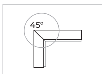
Tok illesztése 45°-ban gérbevágott
