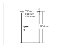
Magyar szabvány méretrend szerint
