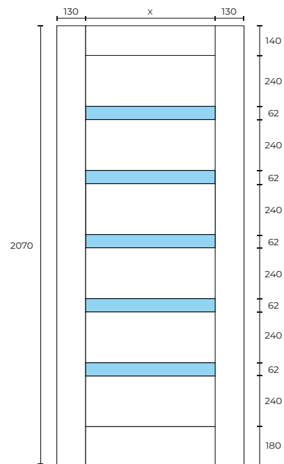
Enzo ajtómodell méretei
