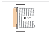
Akár 8 cm-es falvastagsághoz illeszkedő tok
