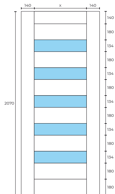
Berg ajtómodell méretei
